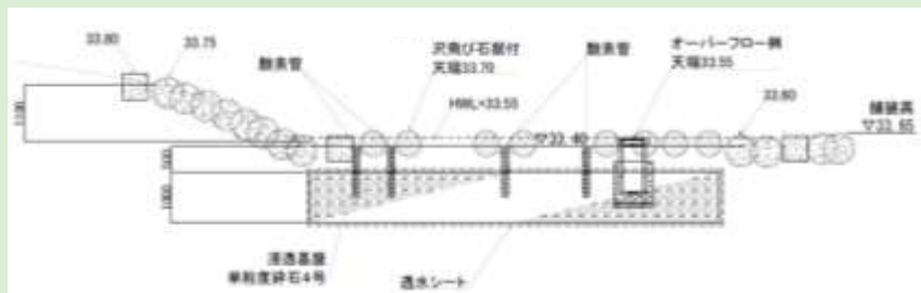
- 断面図 -
