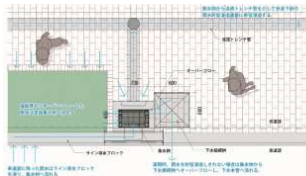
- グリーンインフラシステム概要図 -
