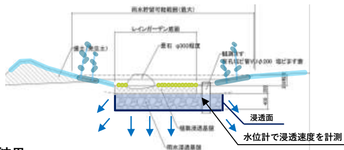
注水試験の実施状況
