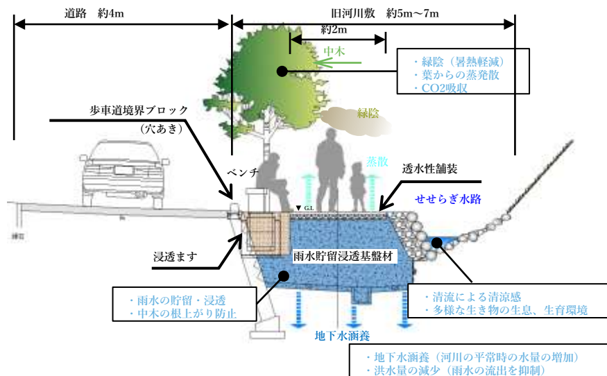
- 断面図 (Cゾーン) -
