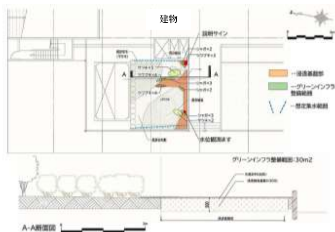
- 竣工図 -
