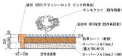
- 断面図 -
